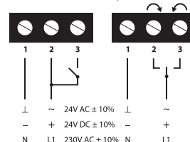
ЭЛЕКТРИЧЕСКОЕ ПОДКЛЮЧЕНИЕ
