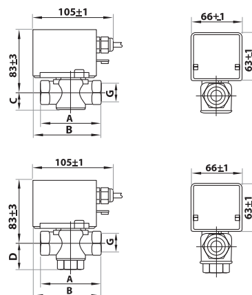
РАЗМЕРЫ (ММ)
