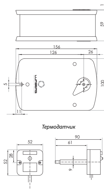
РАЗМЕРЫ (мм)
